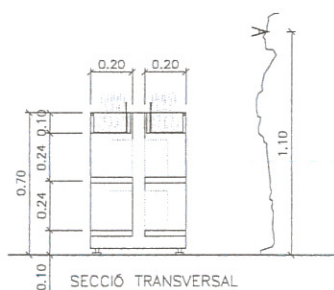
SECCIÓ TRANSVERSAL
