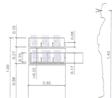
SECCIÓ TRANSVERSAL
