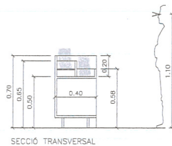
SECCIÓ TRANSVERSAL
