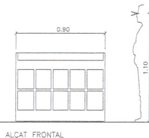
ALÇAT FRONTAL
