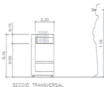
SECCIÓ TRANSVERSAL
