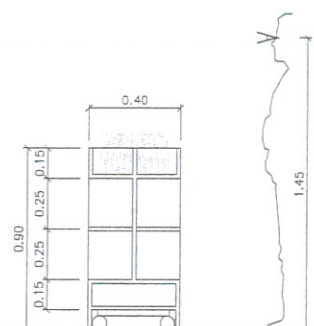
SECCIÓ TRANSVERSAL
