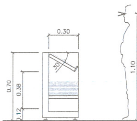
SECCIÓ TRANSVERSAL
