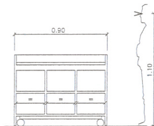
SECCIÓ LONGITUDINAL
