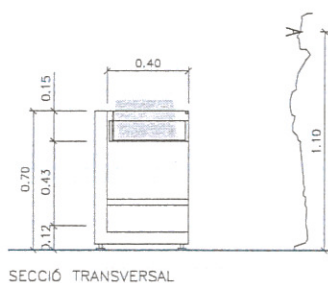
SECCIÓ TRANSVERSAL
