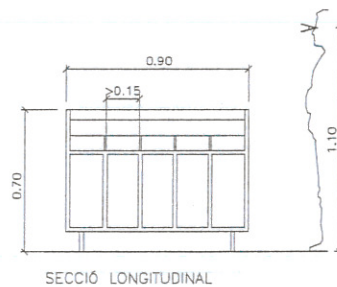
SECCIÓ LONGITUDINAL
