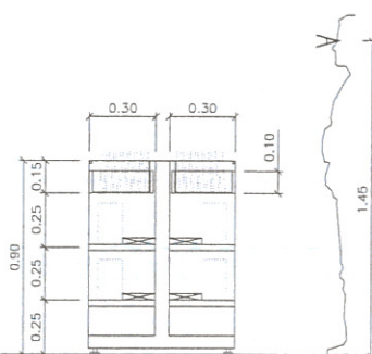
SECCIÓ TRANSVERSAL
