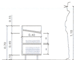
SECCIÓ TRANSVERSAL
