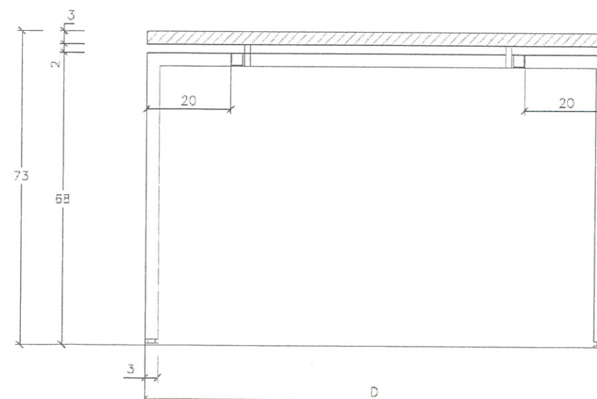
SECCIÓ TRANVERSAL
