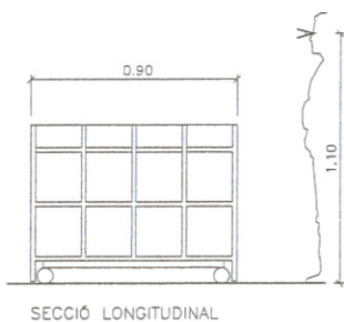
SECCIÓ LONGITUDINAL
