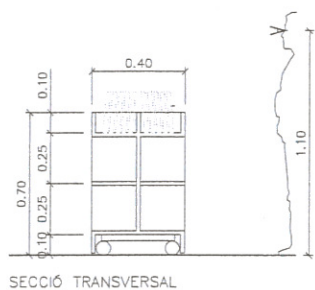
SECCIÓ TRANSVERSAL
