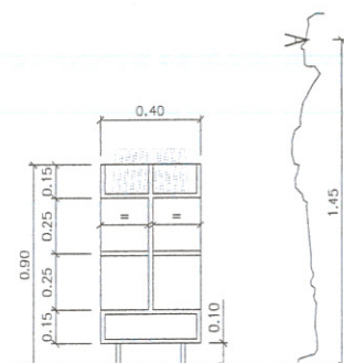
SECCIÓ TRANSVERSAL
