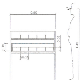
SECCIÓ LONGITUDINAL
