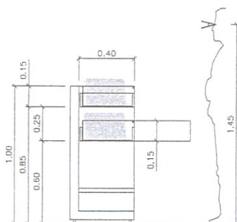
SECCIÓ TRANSVERSAL
