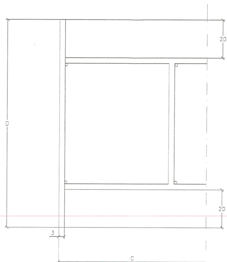
PLANTA
